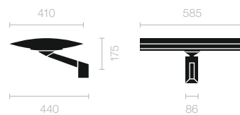
4x 55W Mit Ausleger With bracket
