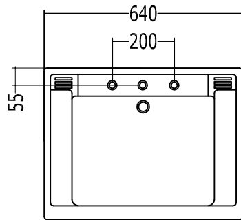
Lavabo con colonna (1-2-3 fori)
