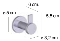
Colgador 1 Robe hook 1 ○ 45.30.01.002 Ⓜ 45.30.01.009
