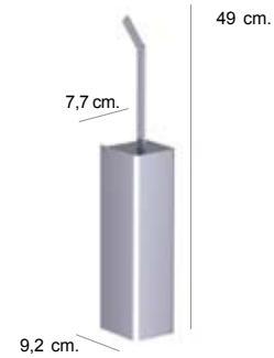
Escobillero suelo Free standing toilet brush
